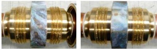
写真12.2-塩水噴霧試験後の供試体
