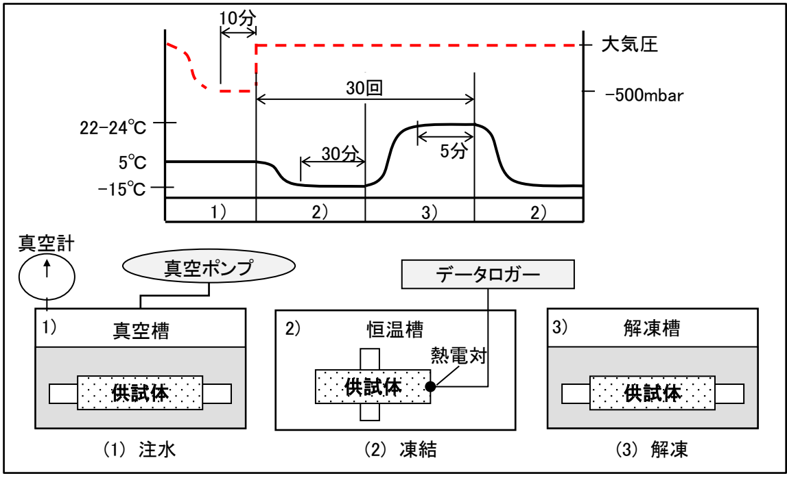
図4-凍結試験
