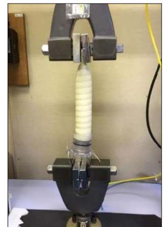
写真4. 引張試験状況
