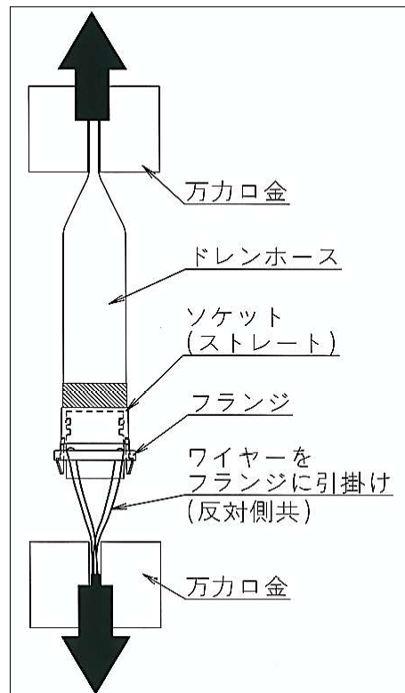
図3. 引張試験
