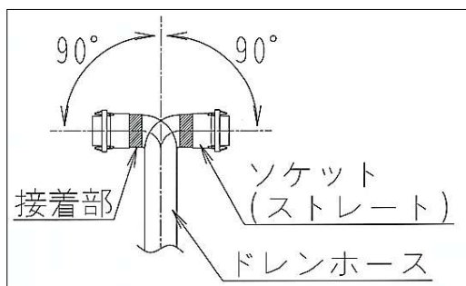
図1. 気密曲げ試験(接着部)
