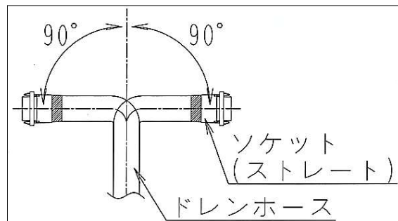
図2. 気密曲げ試験(ホース部)
